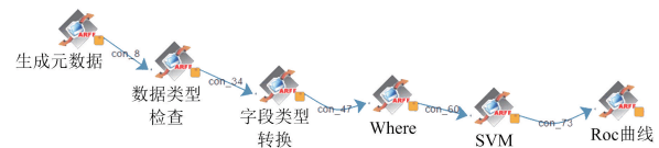
图 5 工作流
